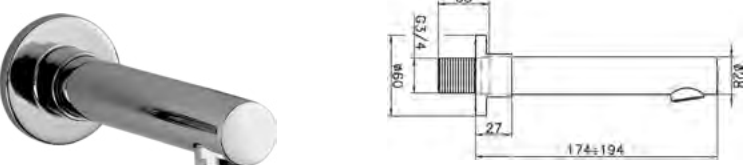
SM 000240 Bocca di Erogazione Filler Spout Bec Verseur
