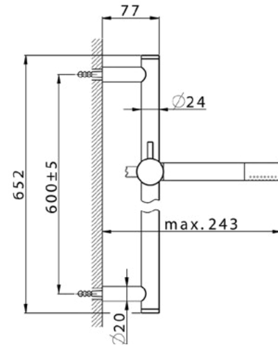
DS 010721 Completo Doccia Saliscendi 60 cm 60 cm Slide Rail Shower Set Ensemble Barre de Douche 60 cm
