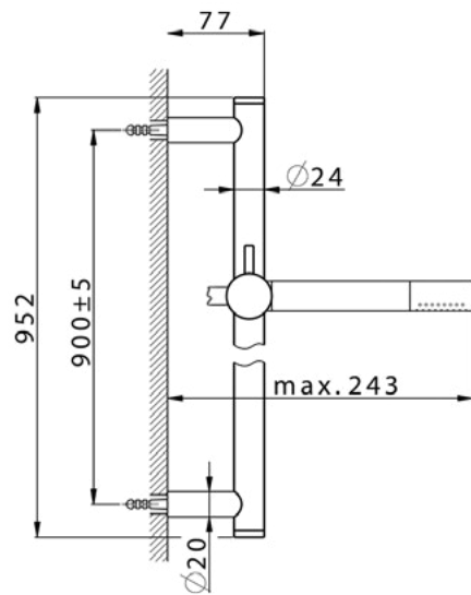
DS 010720 Completo Doccia Saliscendi 90 cm 90 cm Slide Rail Shower Set Ensemble Barre de Douche 90 cm
