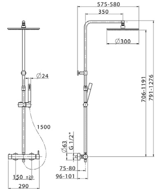
SM 004030 CombiDoccia Monocomando CombiShower Mixer CombiDouche Mitigeur
