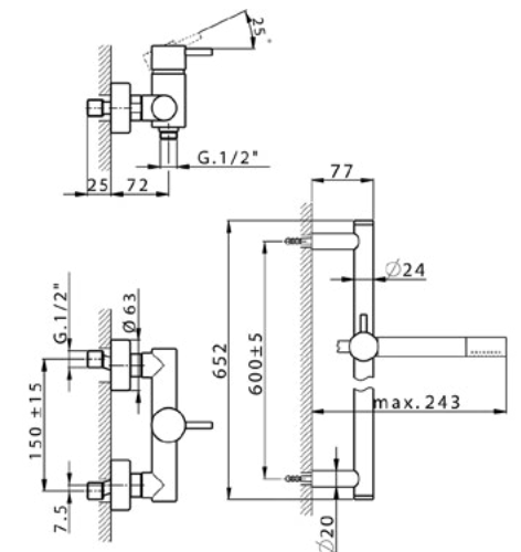
SM 000460 Completo Monocomando Doccia Shower Mixer Set Ensemble Mitigeur Douche
